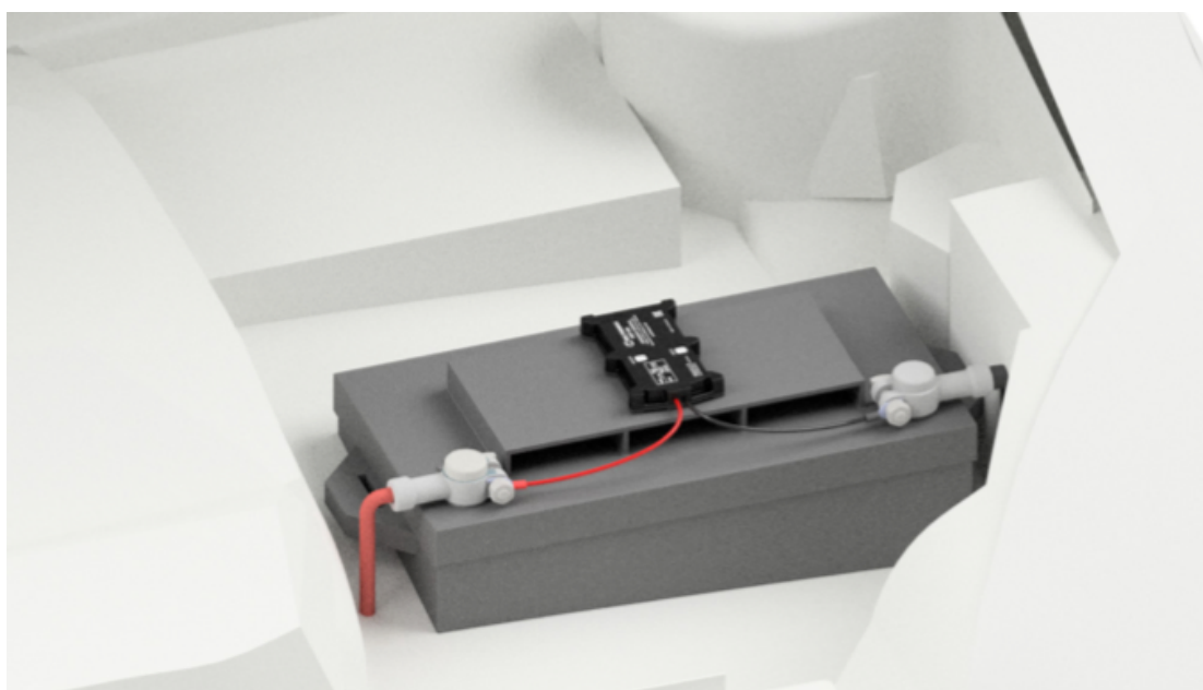
Afbeelding: Voorbeeld van montage van de ACCU GPS Tracker
